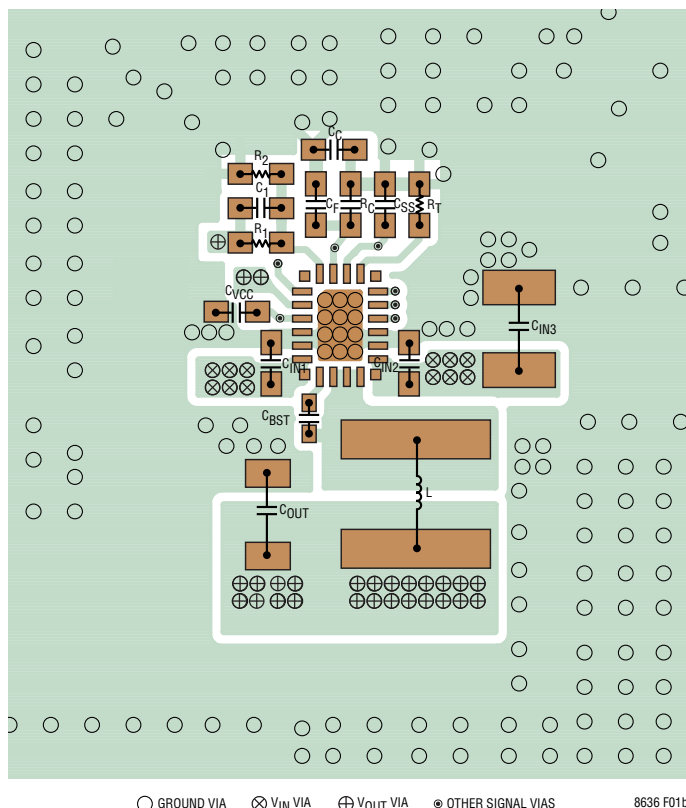
(b) LT8637
