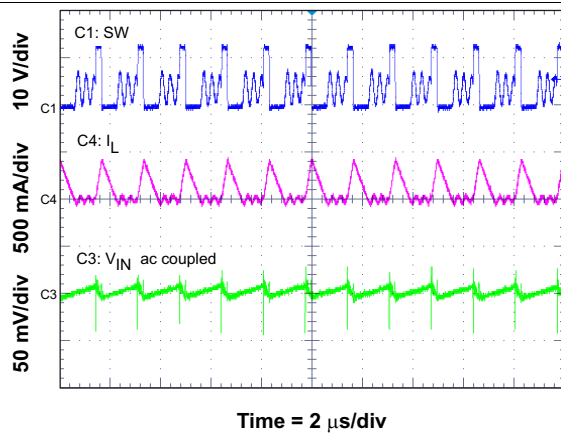
Figure 42. Input Ripple DCM
